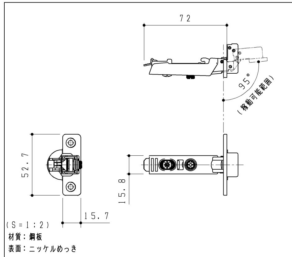
スライド丁番（キャッチなし）（2ヶ）
