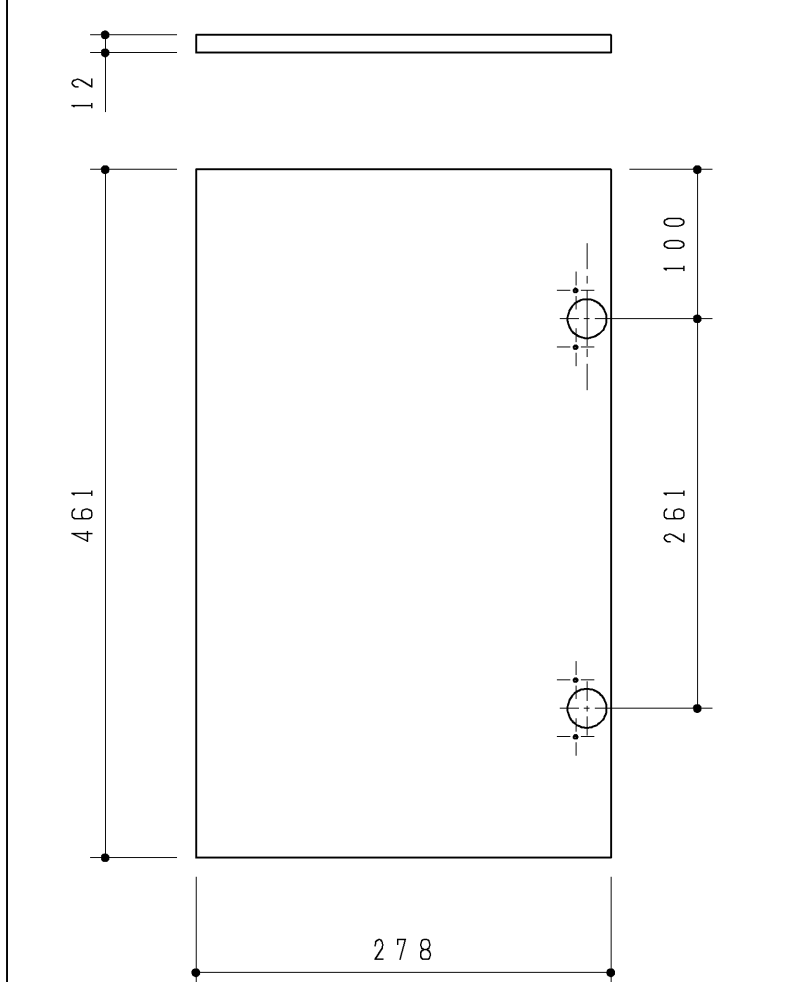
丁番用スペーサー（2ヶ）
