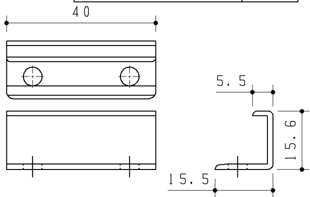
キャップセット
