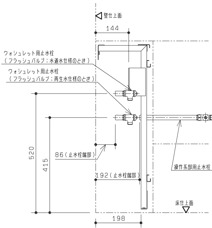
Q 視図
