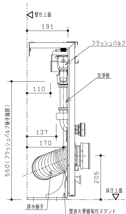
P 視図
