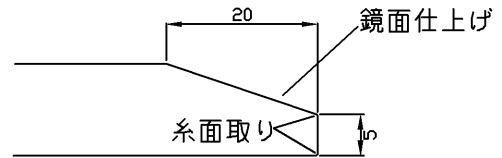
B部（テーパー部）拡大図
