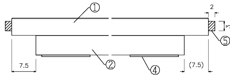
A-A断面図
