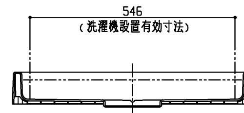
断面B-B
