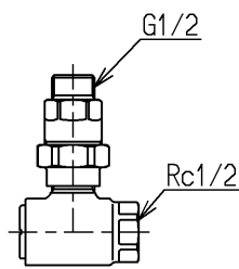
止水栓部(2ヶ)
