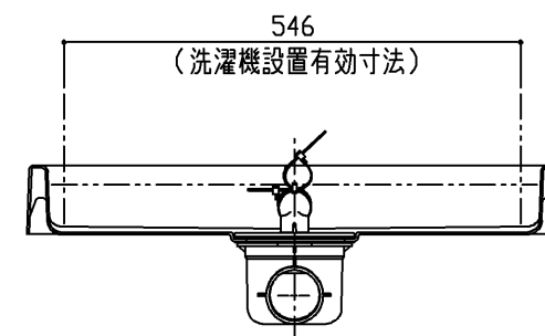
断面B-B
