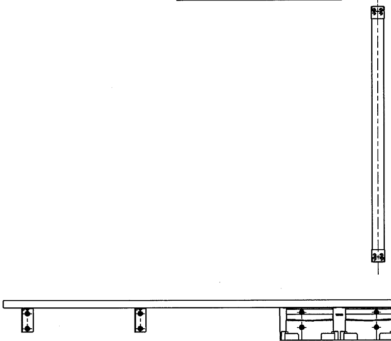
左壁設置の場合(1:10)
