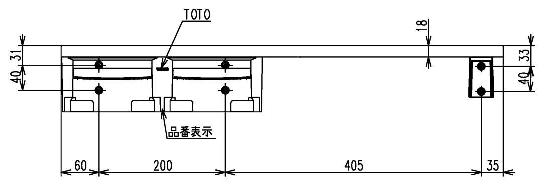
左壁設置の場合
