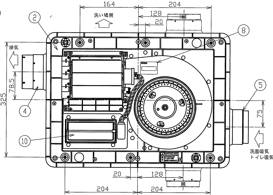
天井取付図 (1:5)
