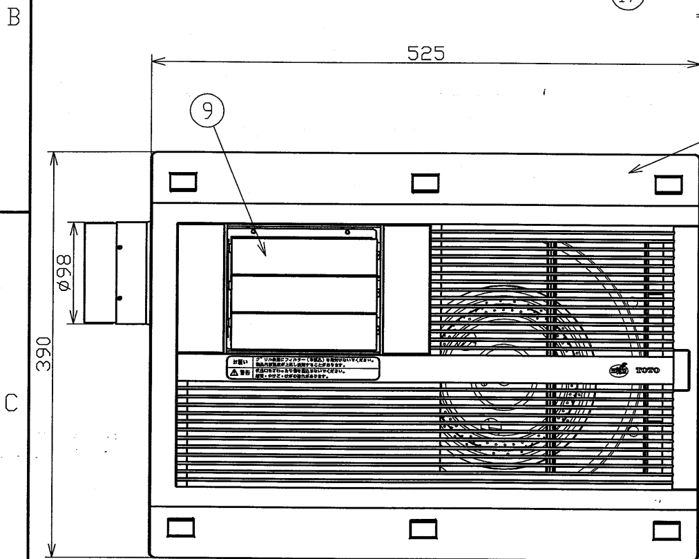
天井取付図 (1:5)
