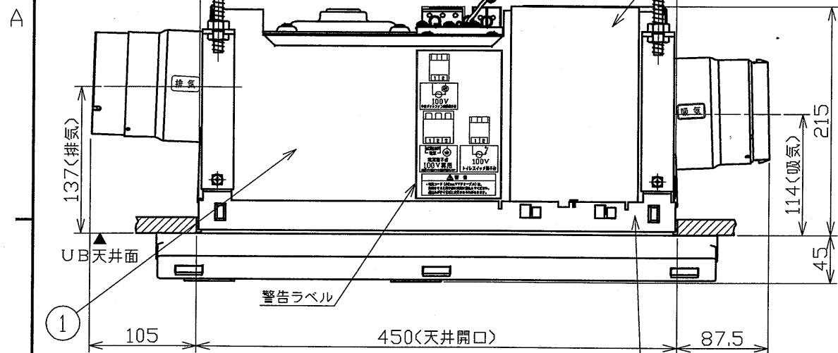
天井取付図 (1:5)
