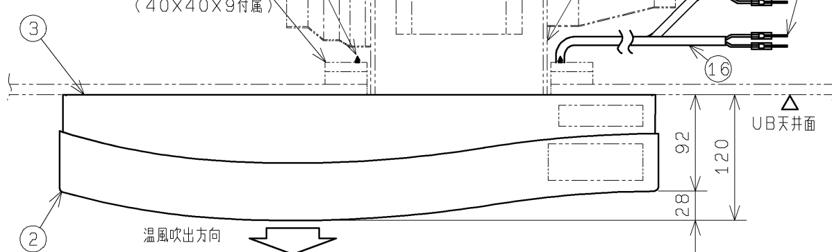
天井取付図
