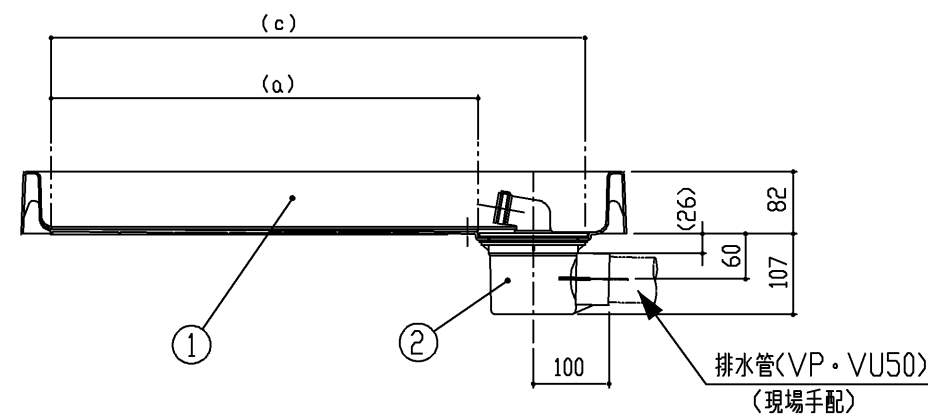
断面A-A
