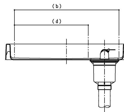
断面B-B
