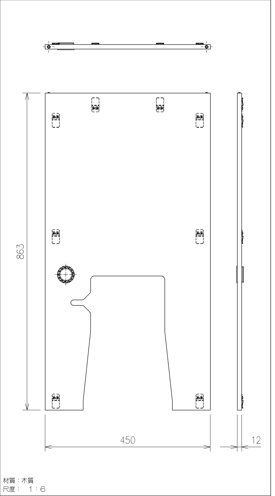
前板組品
