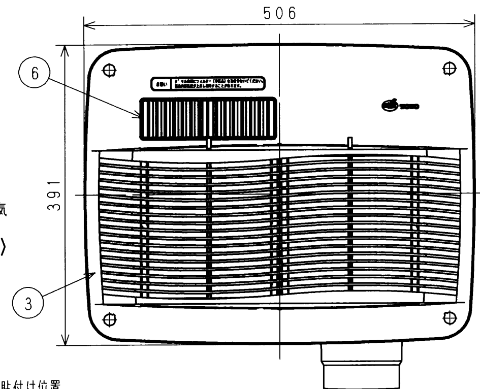
天井取付図 (1:5)
