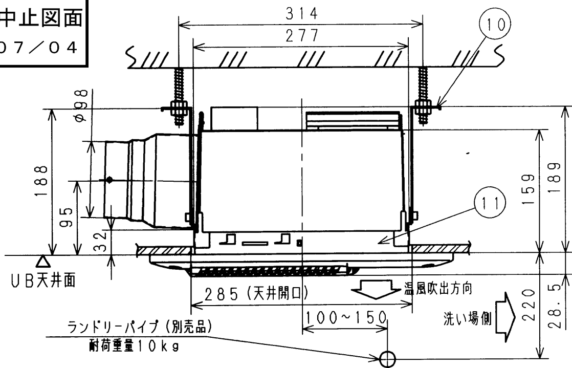
天井取付図 (1:5)
