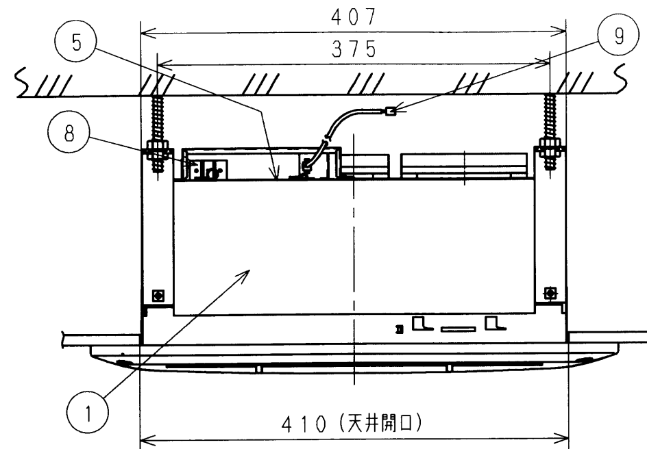
天井取付図 (1:5)
