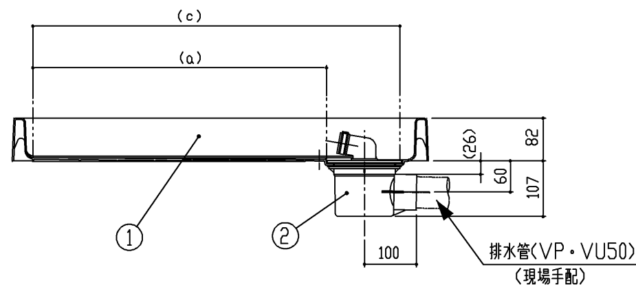
断面A-A
