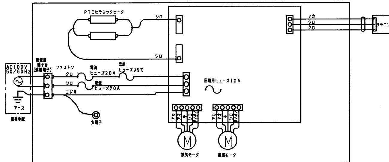
浴室換気暖房乾燥機 本体
