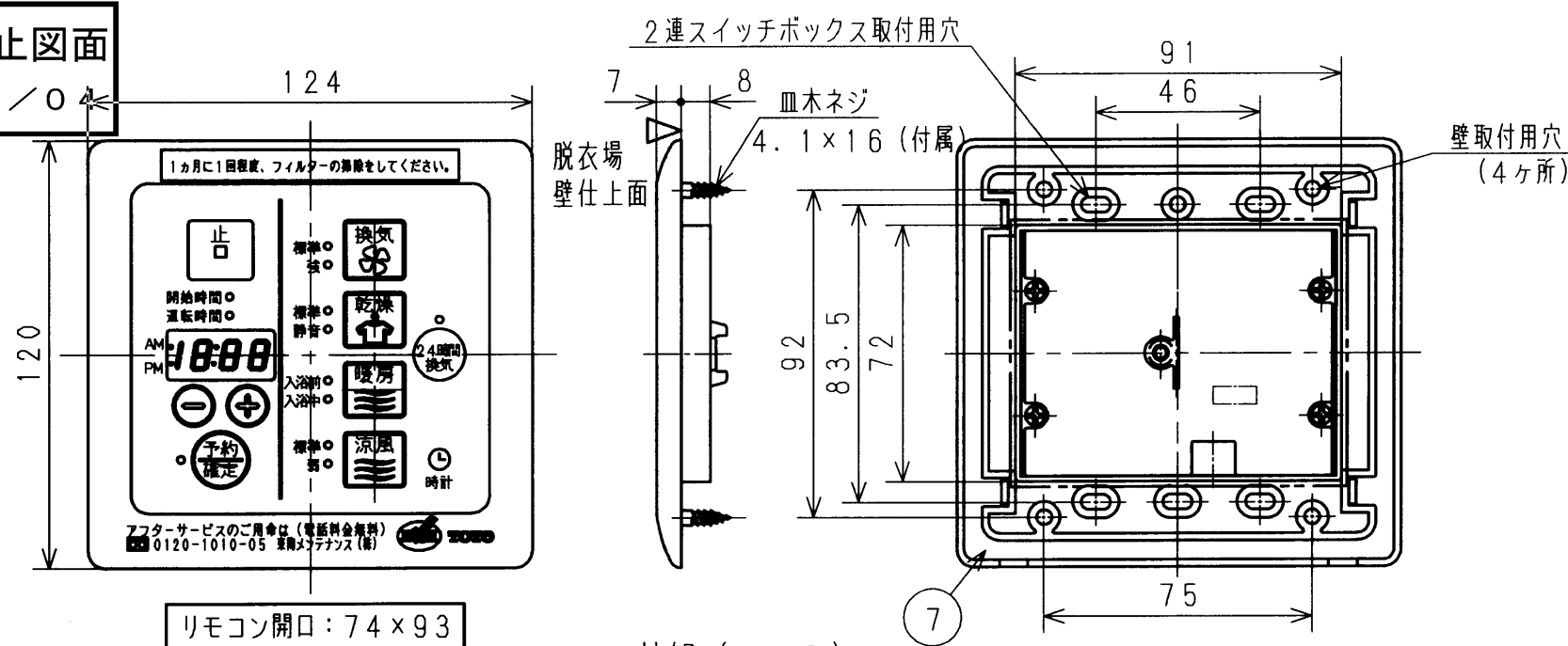
リモコン外観 (1:2)
