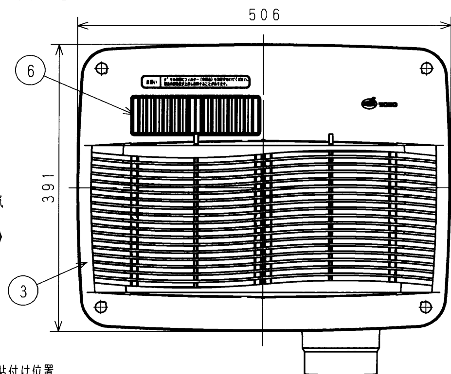
天井取付図 (1:5)
