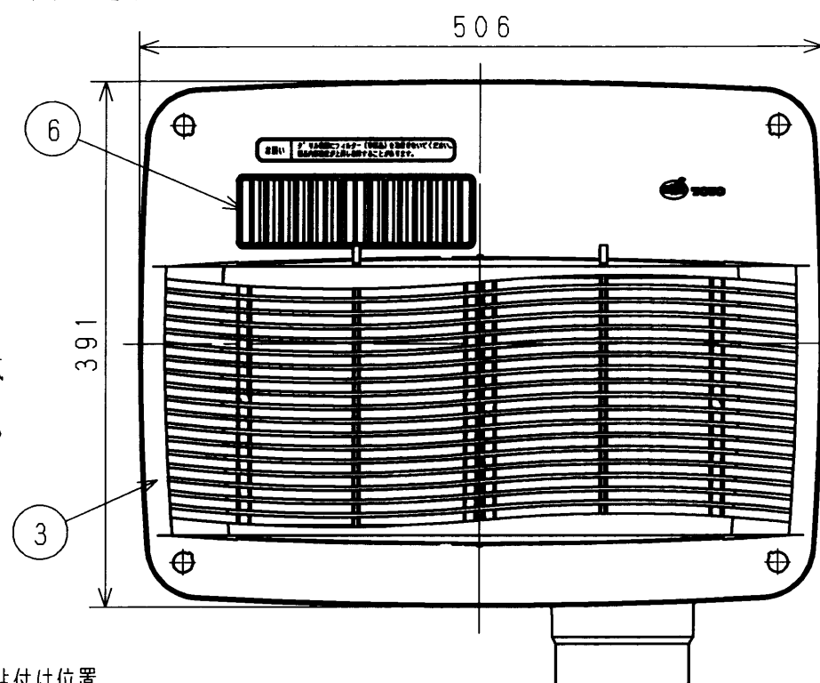
天井取付図 (1:5)
