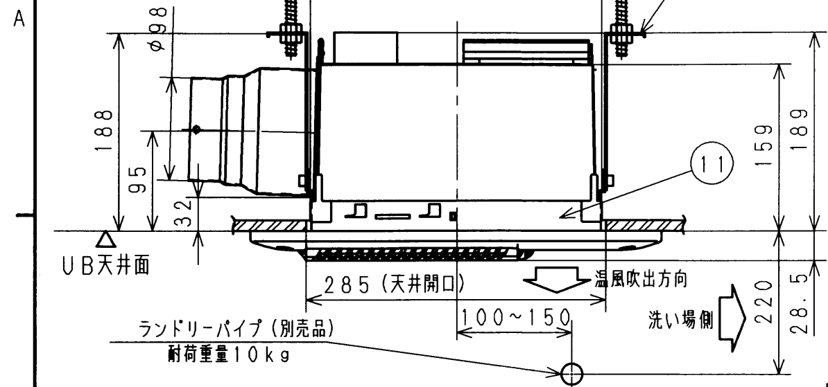
天井取付図 (1:5)
