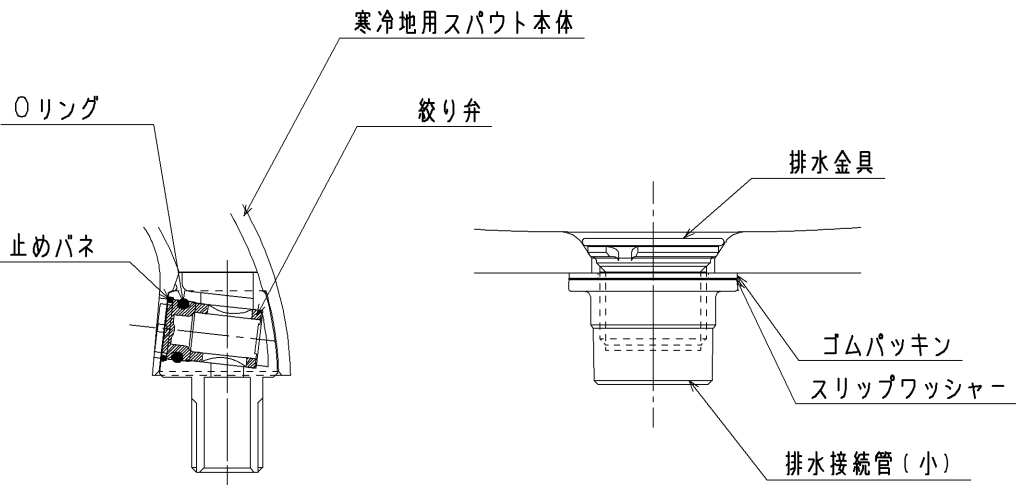
E-E断面詳細図 (S=1:1)
