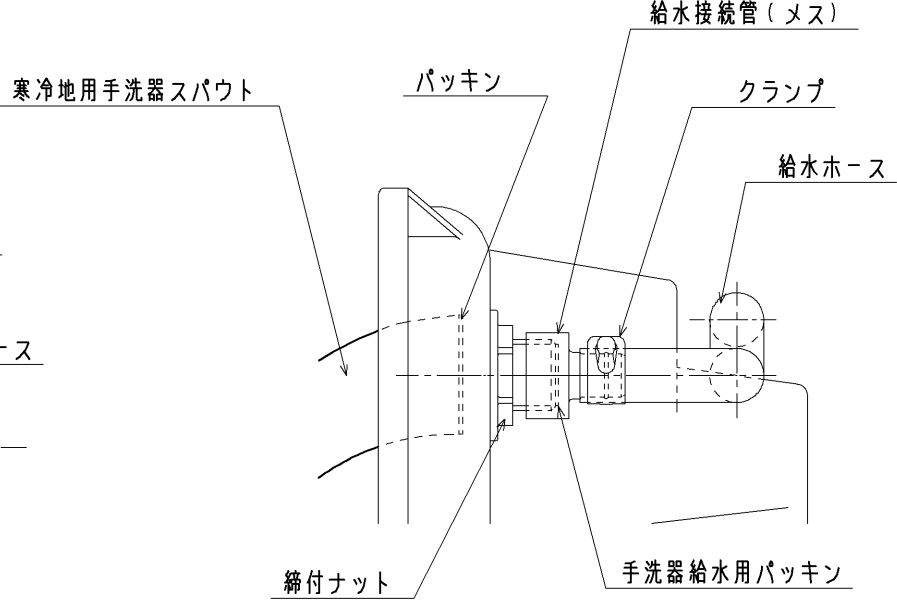
D部詳細図 (S=1:1)
