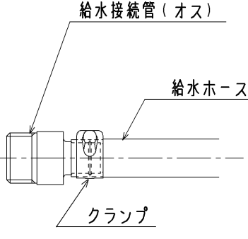
C部詳細図 (S=1:1)
