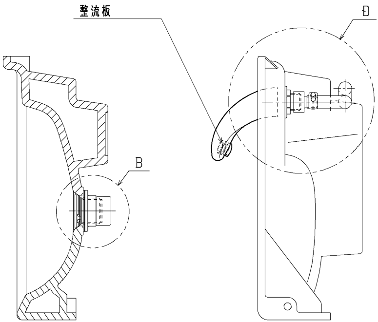
A-A断面詳細図
