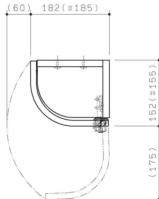
開口状態図
