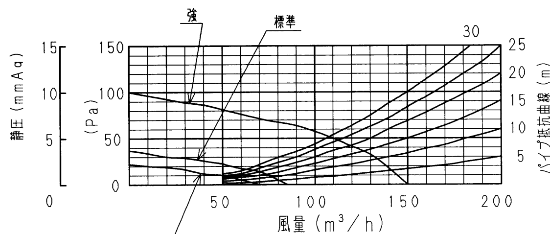
靜壓風量特性曲線
