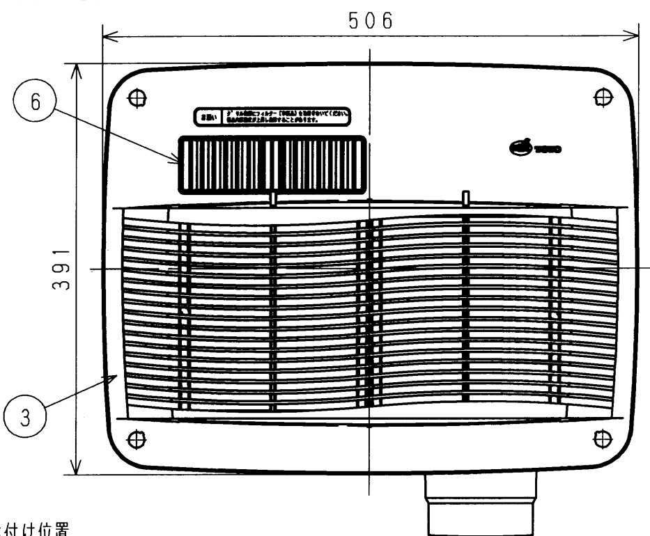
天井取付図 (1:5)
