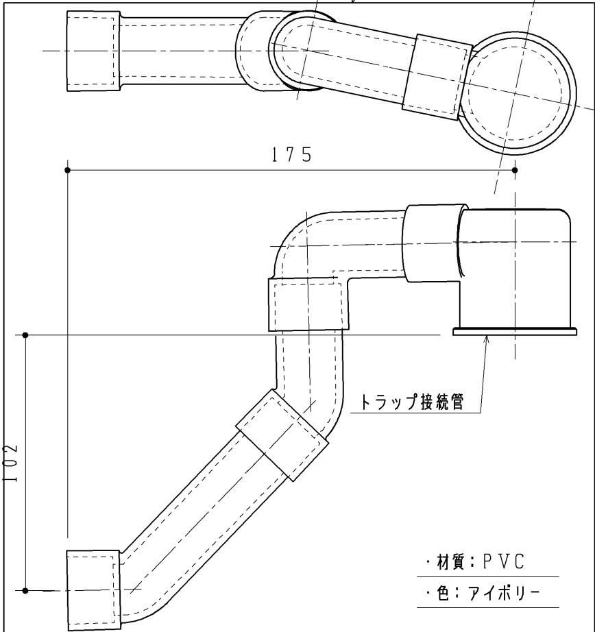
手洗排水ホースセット (床排水)
