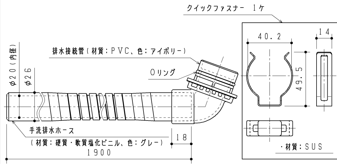
手洗排水ホースセット (床排水)
