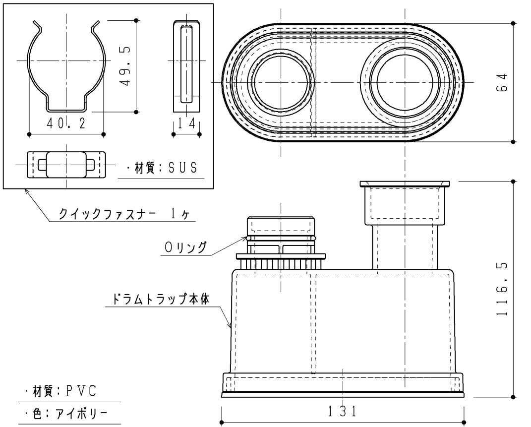
排水金具セット
