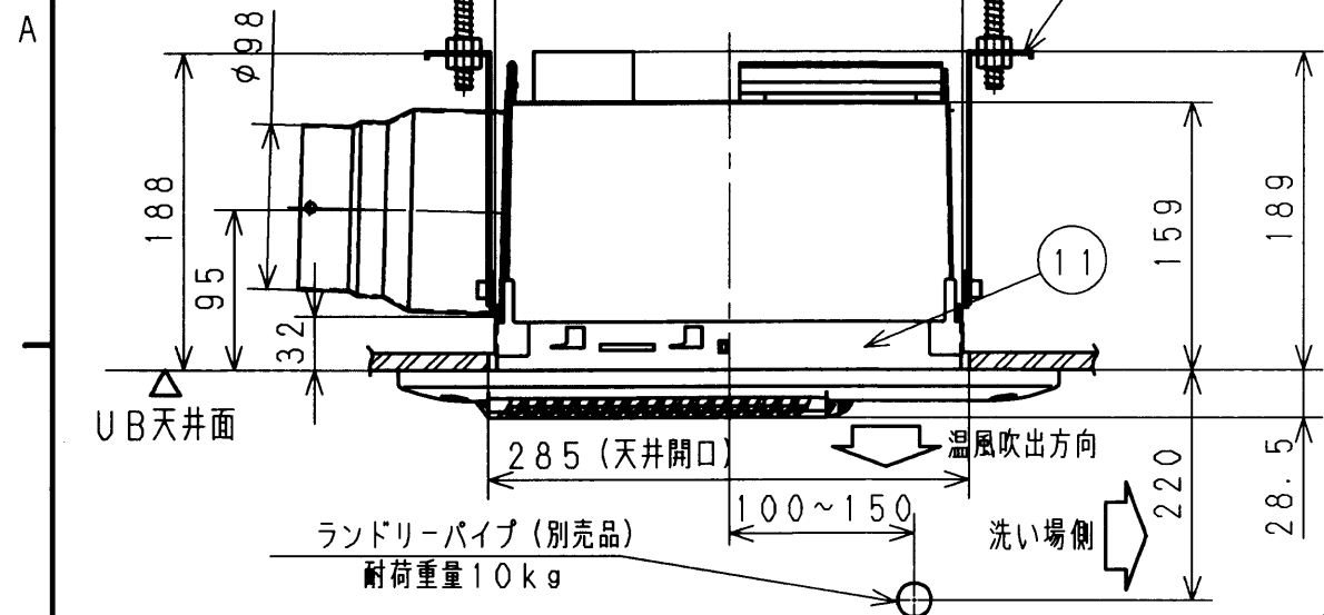
天井取付図 (1:5)
