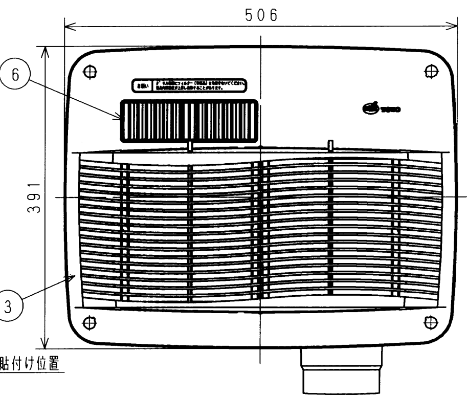
天井取付図 (1:5)
