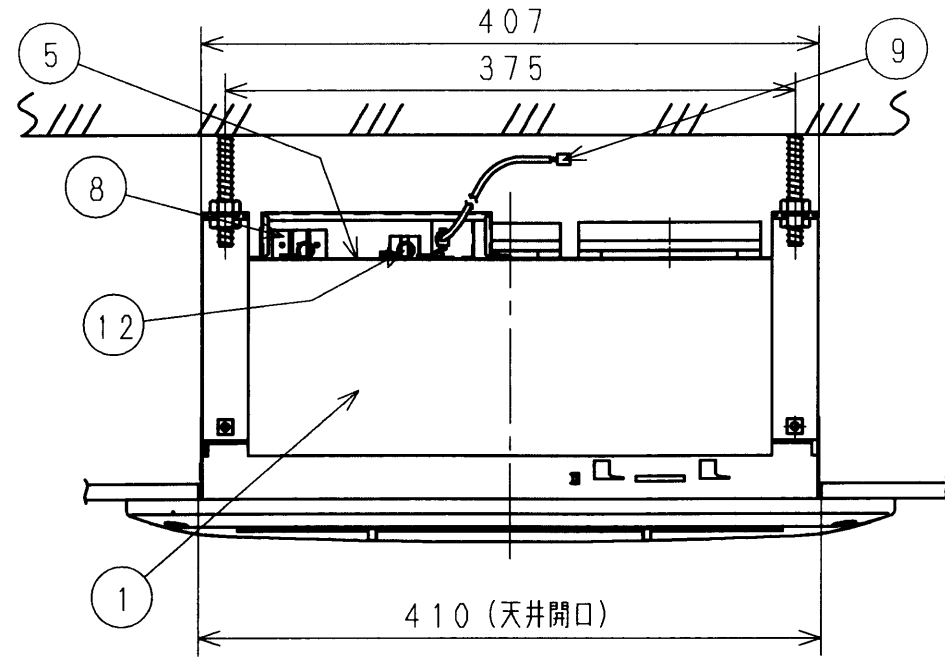
天井取付図 (1:5)
