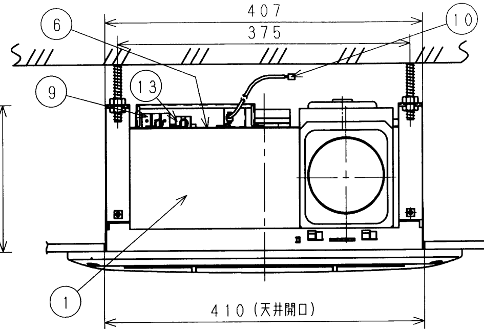
天井取付図 (1 : 5)
