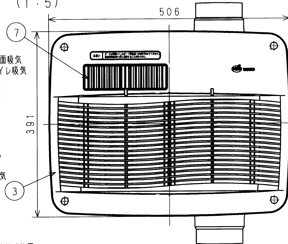
天井取付図 (1 : 5)
