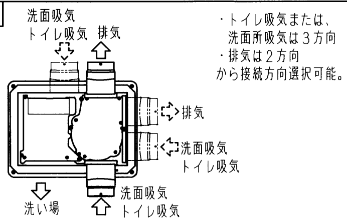
天井裏から見た図
