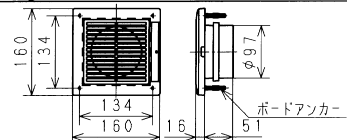
⑭ 吸込ログリル
