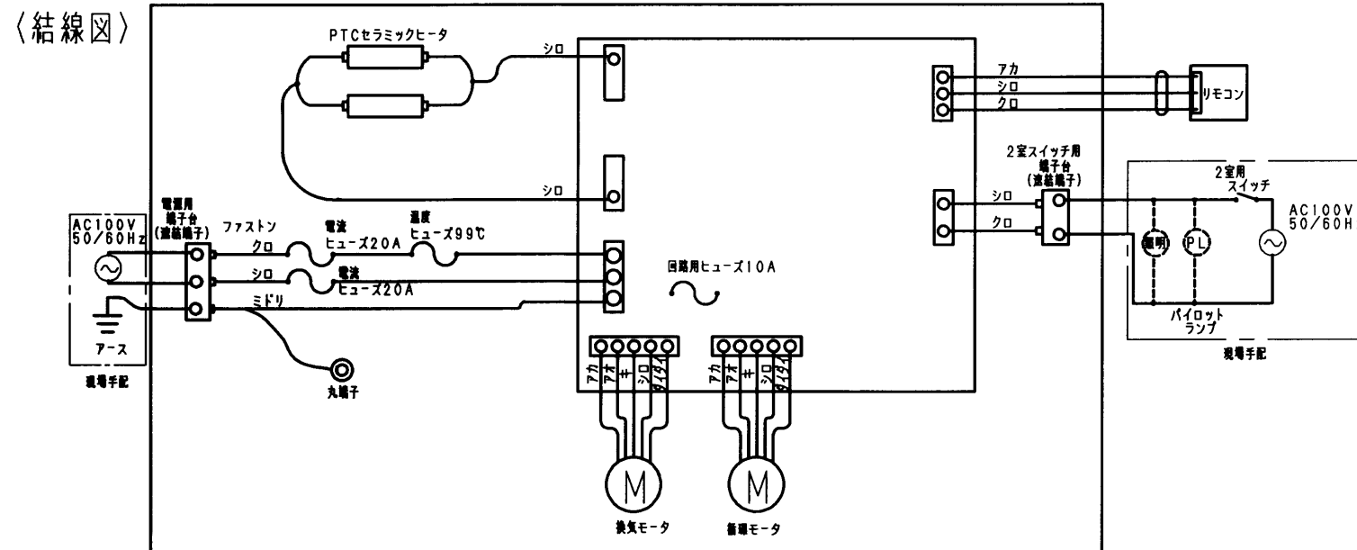
浴室換気暖房乾燥機 本体
