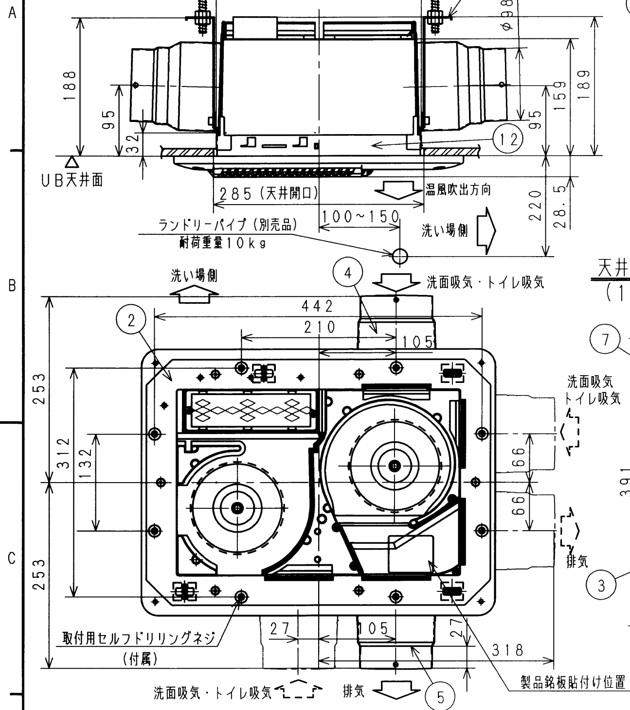
天井裏から見た図
