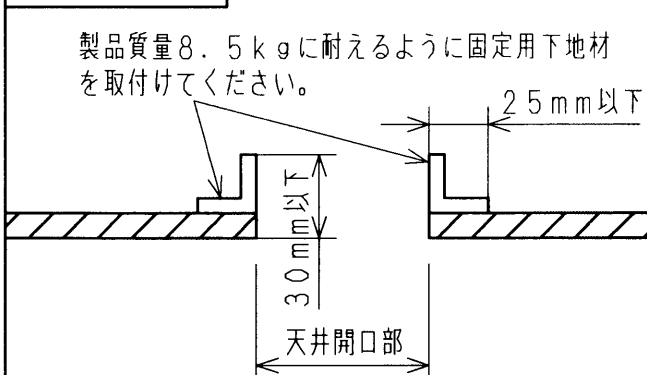
天吊りしない場合
