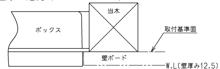
① 壁厚み12.5 (スペーサーなし)
