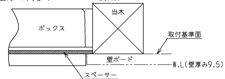
② 壁厚み9.5 (スペーサー使用)
