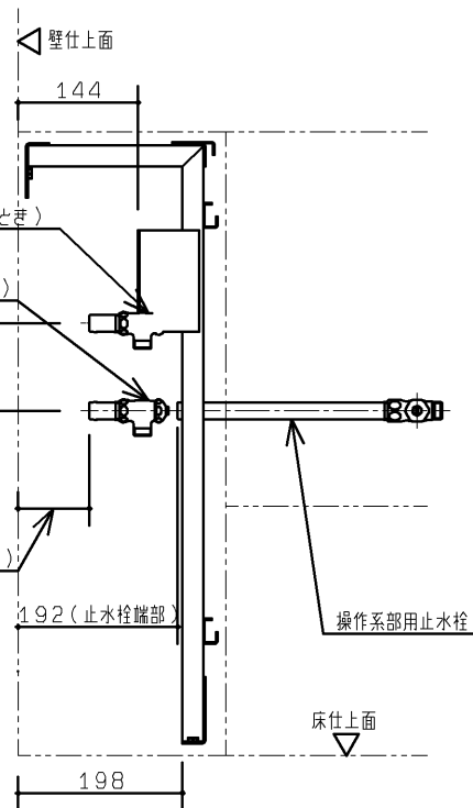
Q 視圖
