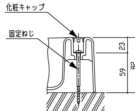
固定部詳細(尺度フリー)
