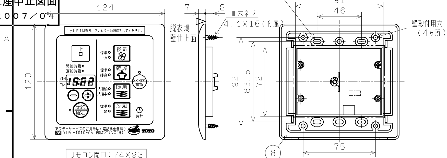
リモコン外觀(1:2)
