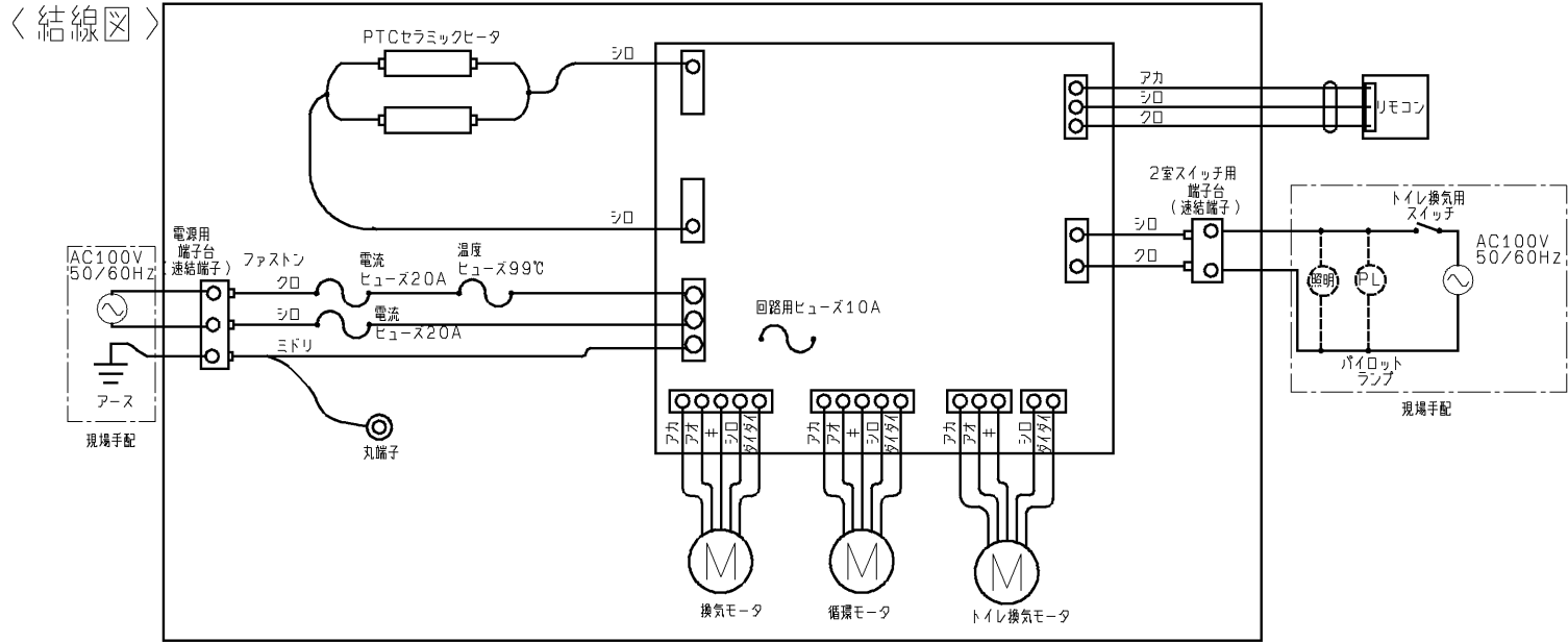
浴室換気暖房乾燥機 本体
