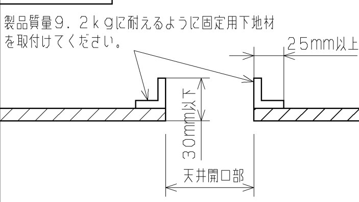
天吊りしない場合
