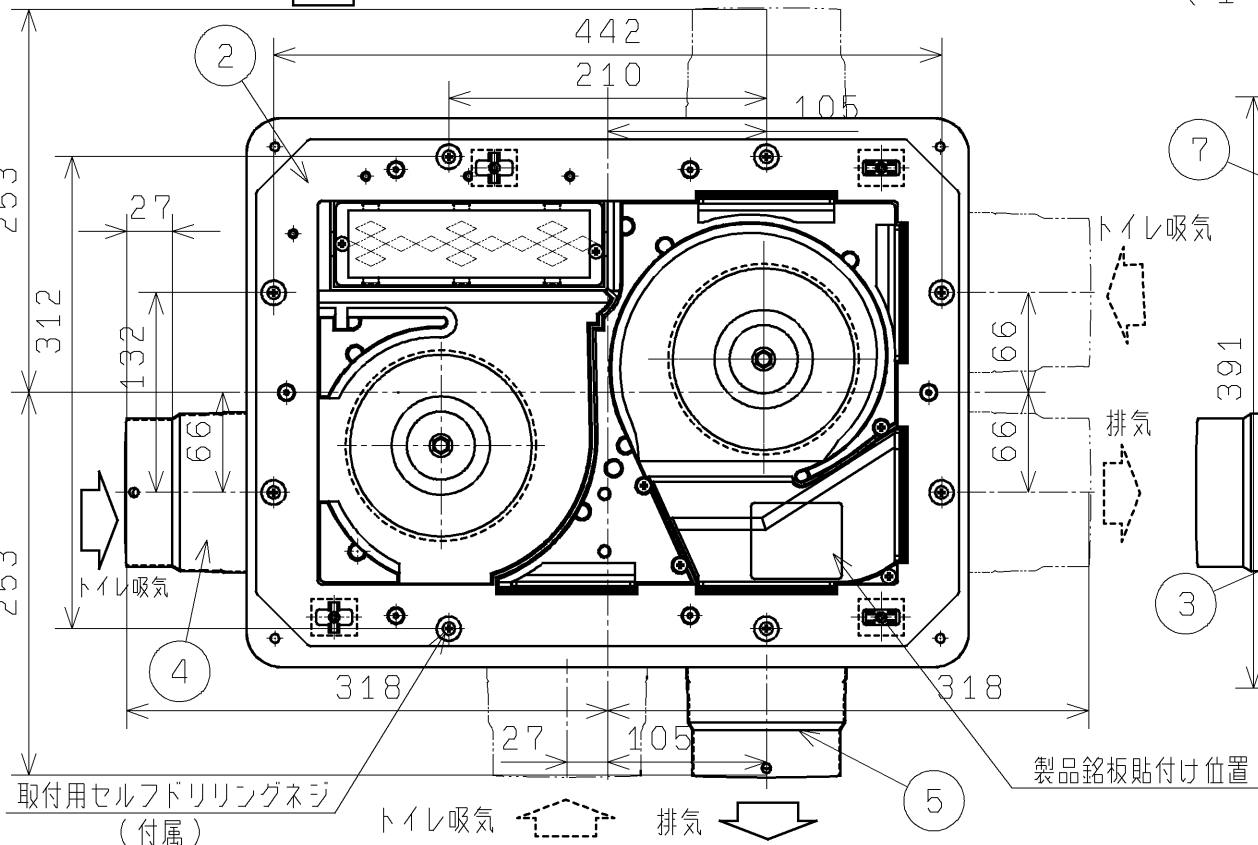
天井裏から見た図
