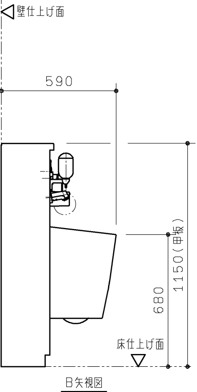
B矢視図
