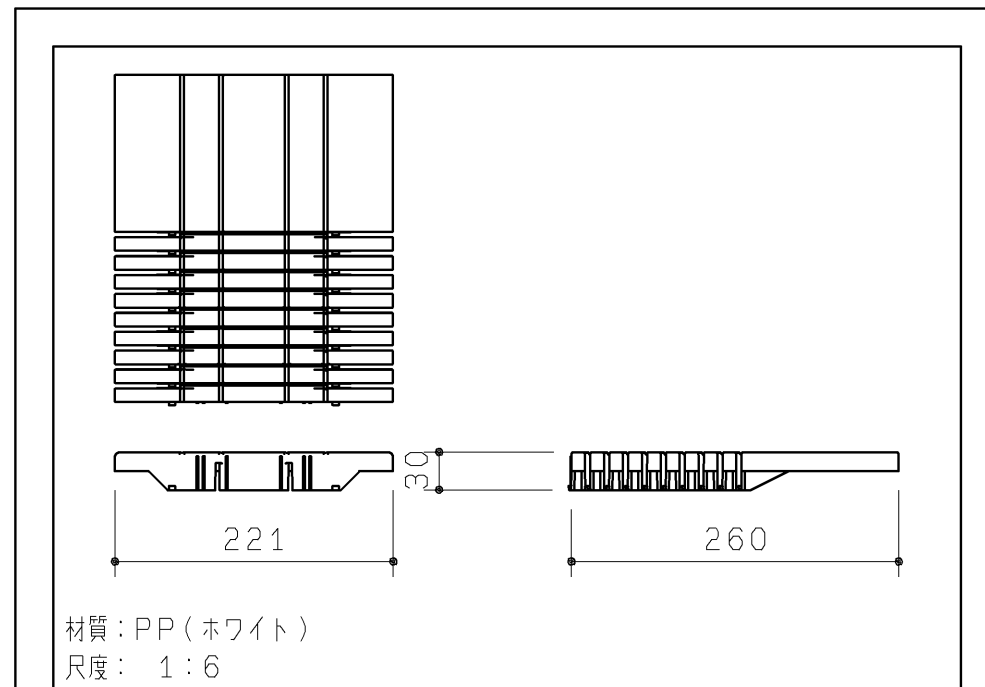
棚板(2ヶ)
