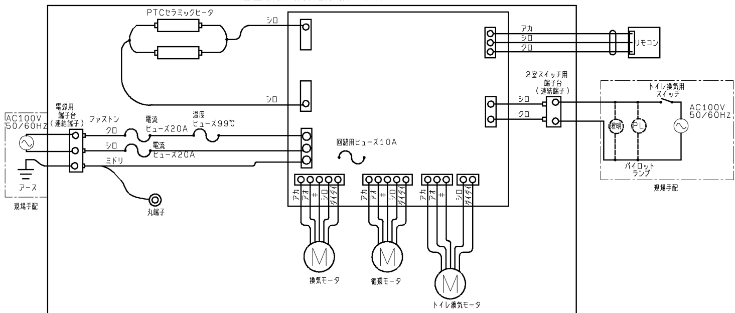
〈結線図〉 浴室換気暖房乾燥機 本体
