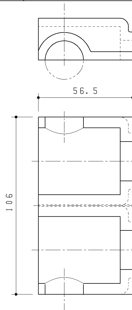
防露カバー（分岐金具部）
