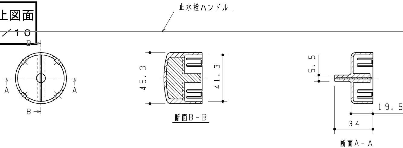
止水栓ハンドル取付材
