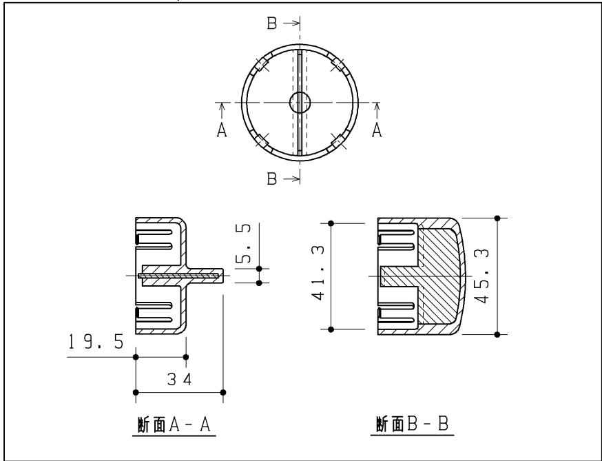
止水栓ハンドル取付材
