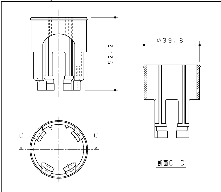
止水栓ハンドル取付材
