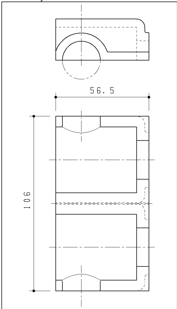
防露カバー（止水栓用）
