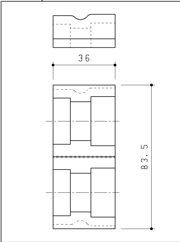
防露カバー（分岐金具部）
