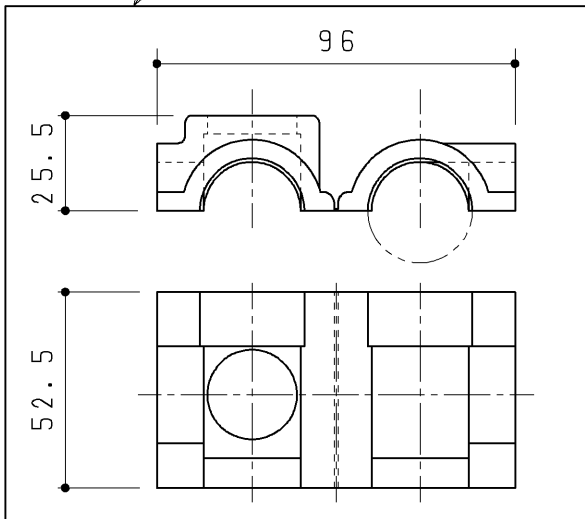
防露カバー（分岐金具部）
