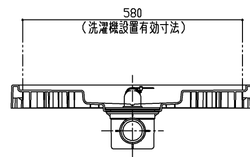
断面B-B
