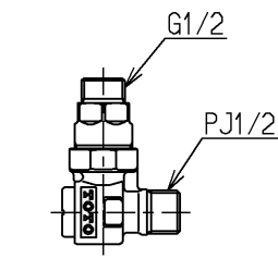
止水栓部 (2ヶ)
