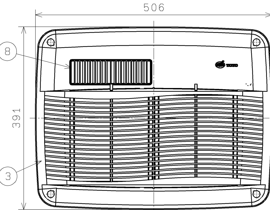
天井取付図 (1:5)
