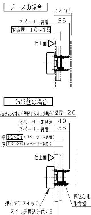
押しボタン断面詳細図 (S=1:5)
