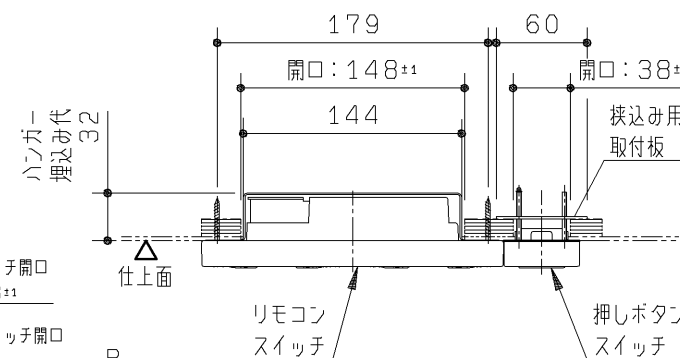
B-B断面詳細図 (S=1:5)
