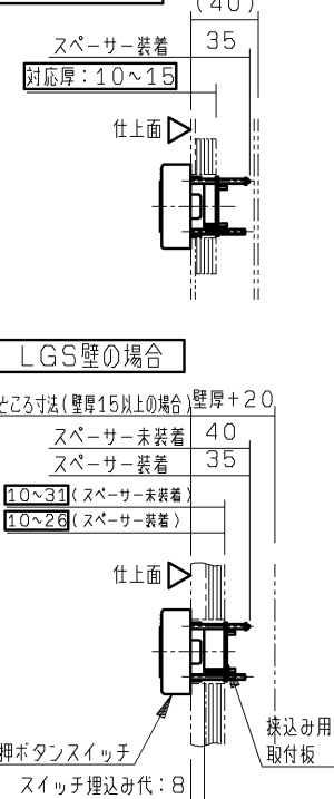
押しボタン断面詳細図 (S=1:5)
