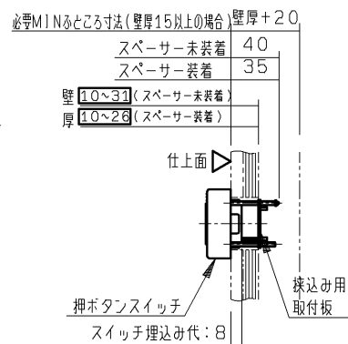
押しボタン断面詳細図 (S=1:5)
