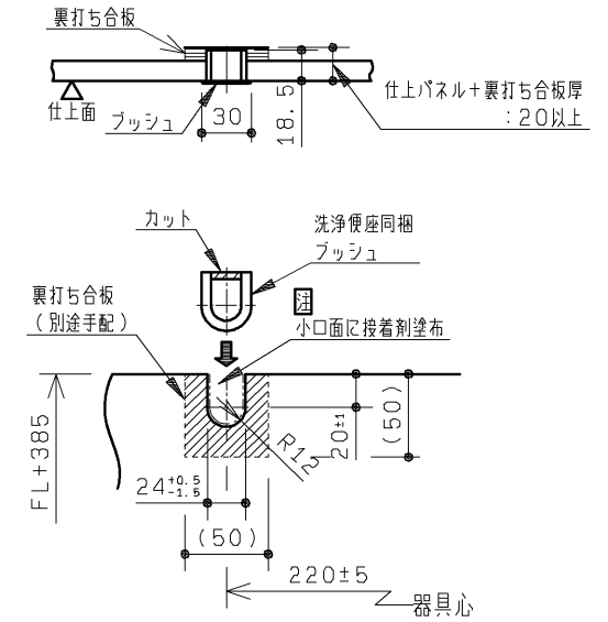
A部詳細図 (S=1:5)
