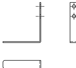
付属部品\詳細図 (1:3)
