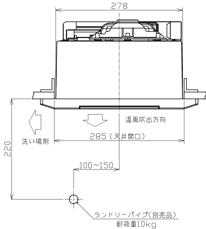
A-A断面
