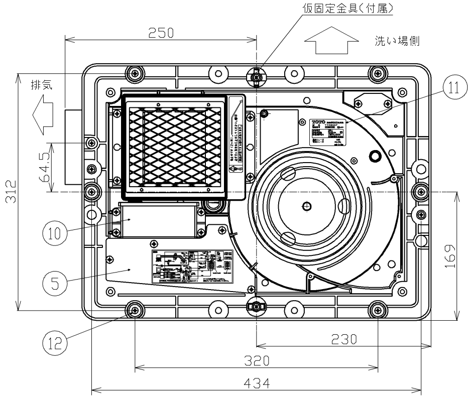
天井取付図 (1:5)
