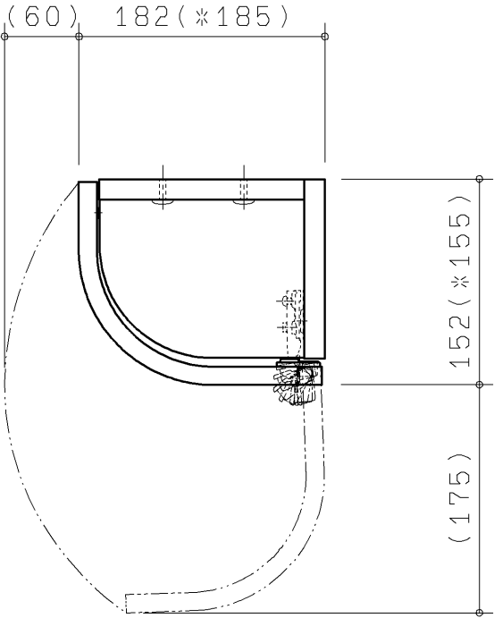
開口状態図
