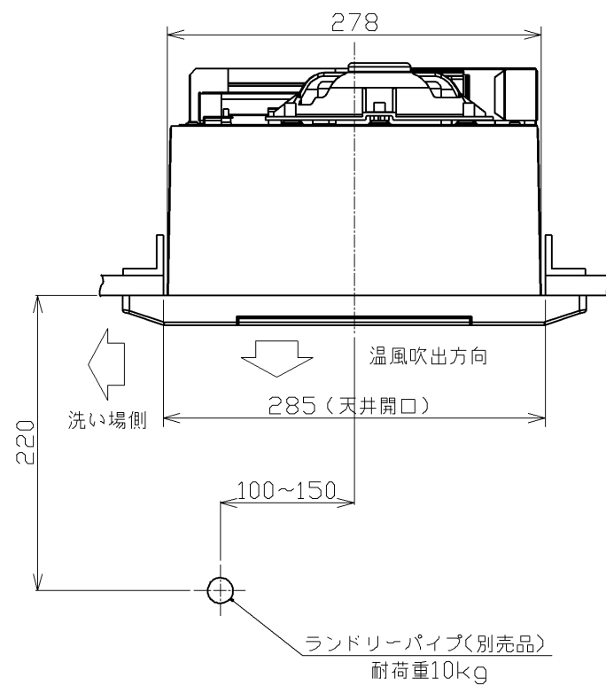
A-A断面
