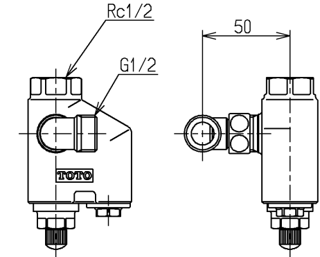
止水栓部(2ヶ入り)
