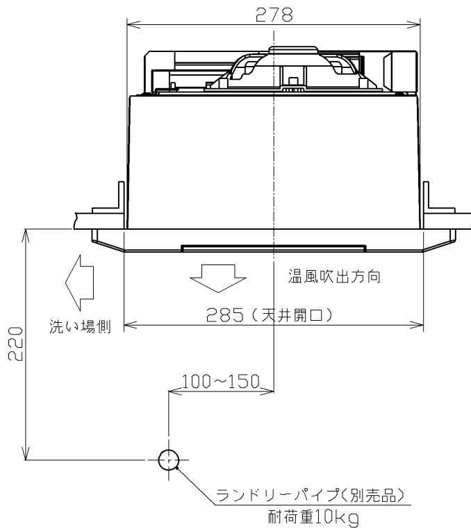
A-A断面
