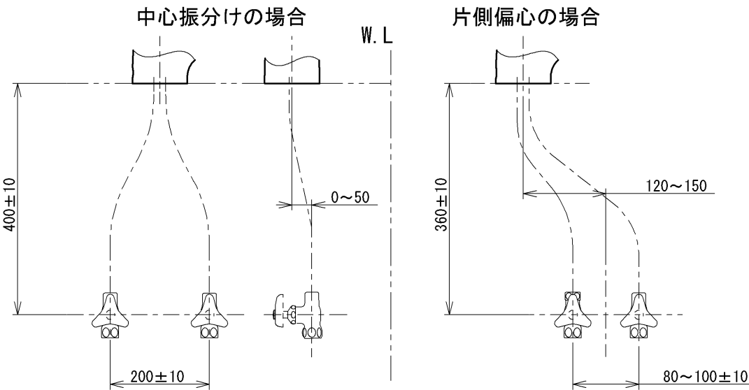
止水栓推奨取付位置
