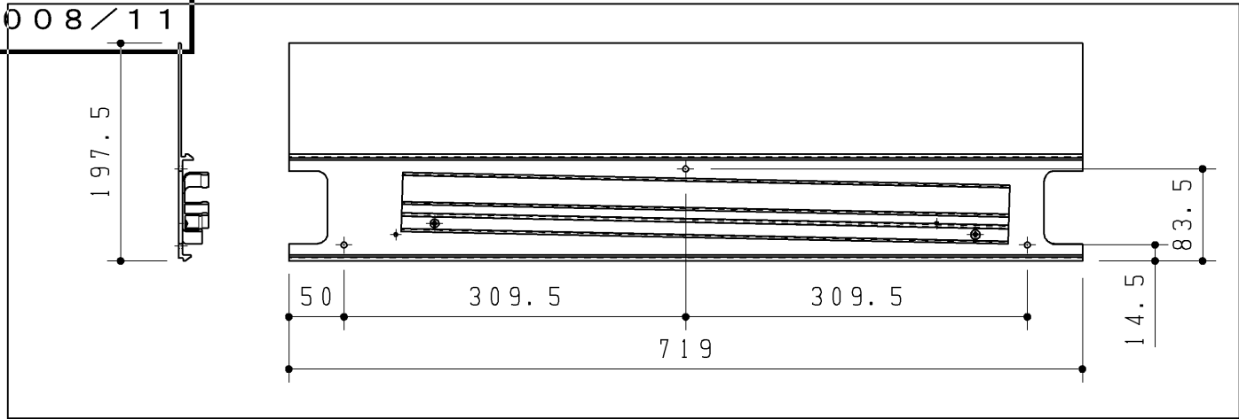
配管カバー
