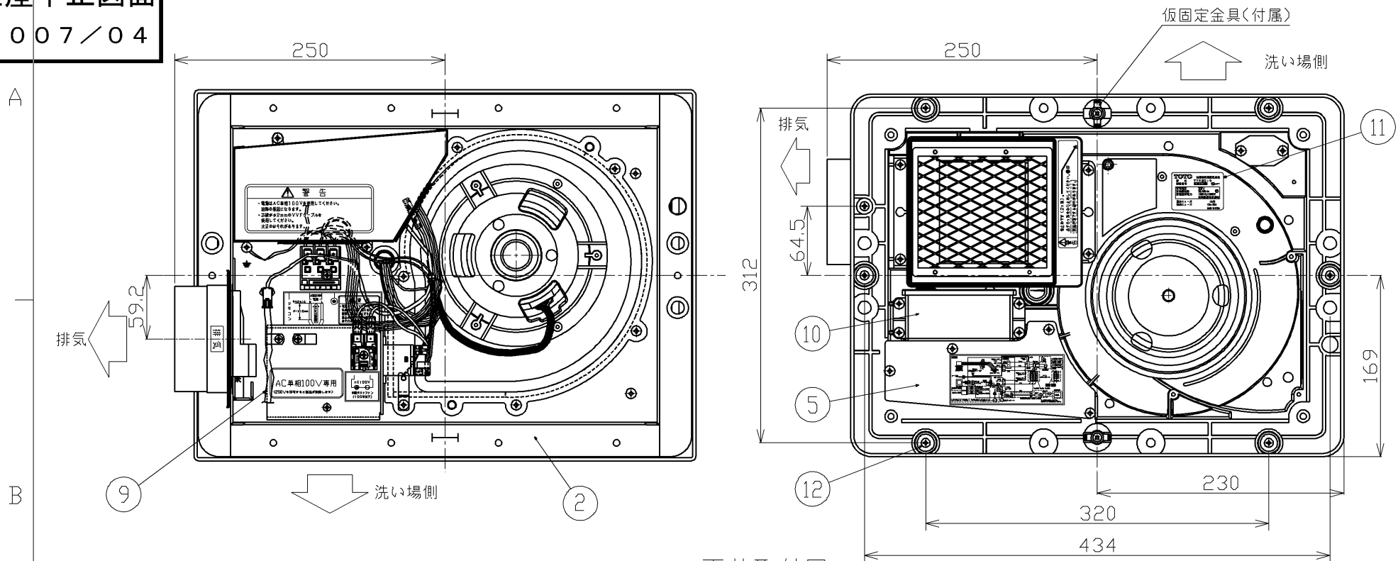
天井取付図 (1:5)
