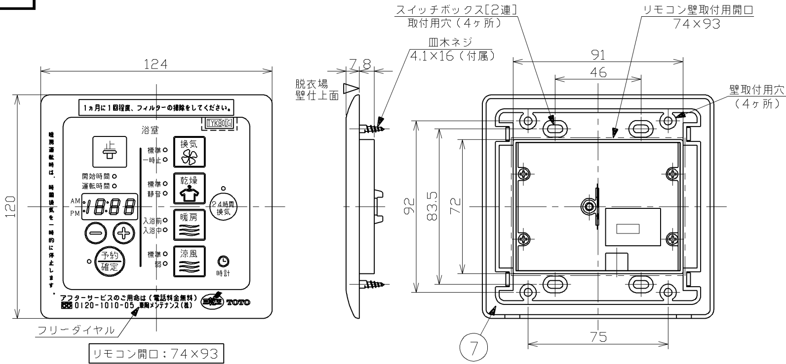
リモコン外観 (1:2)
